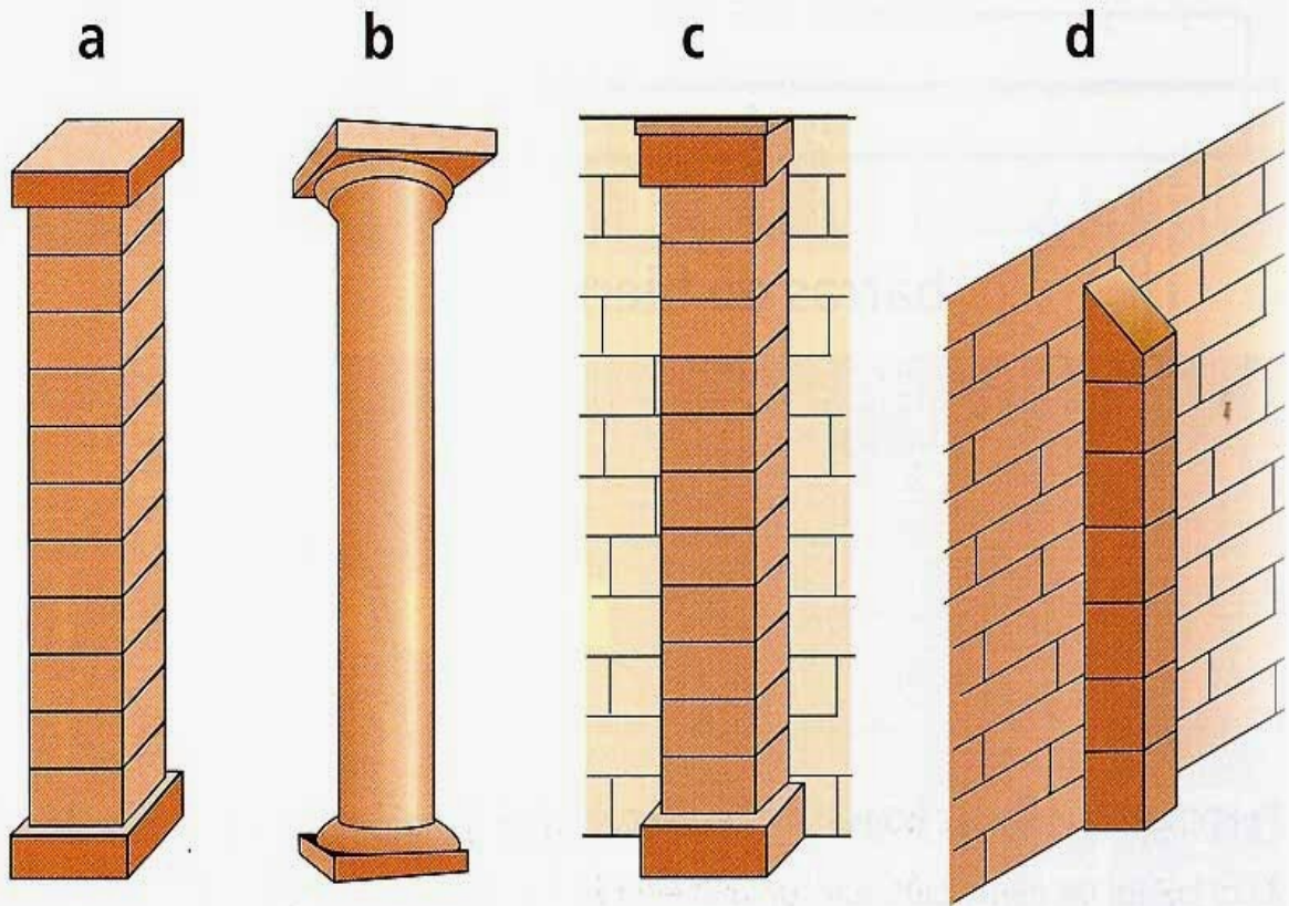
▲ Imagen 14. Pilares y columnas: a) pilar, b) columna, c) pilastra, d) estribo o contrafuerte.
